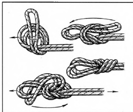
Двойной проводник (заячьи ушки)
