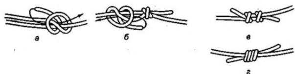
Узел «грейпвайн»
